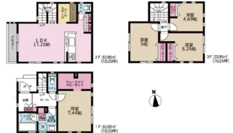
間取図
