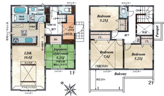
1号地間取図
